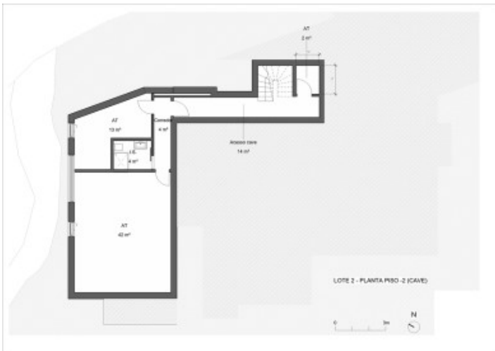
Floorplan Lote 2 -2
